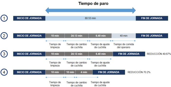
Figura 14. Actividades antes y después de la mejora SMED
