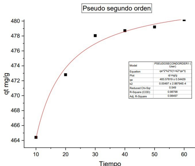
Gráfica 10. Pseudo segundo orden
