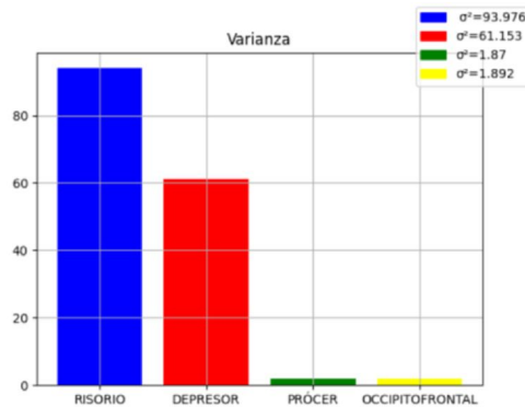
Figura 8. Gráfica de barras de la varianza
