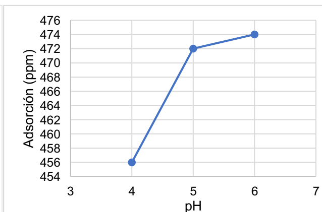
Gráfica 9. Efecto del pH en la adsorción de NM
