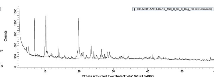
Gráfica 3. Difractograma de polvos cristalinos posterior a la remoción de NM
