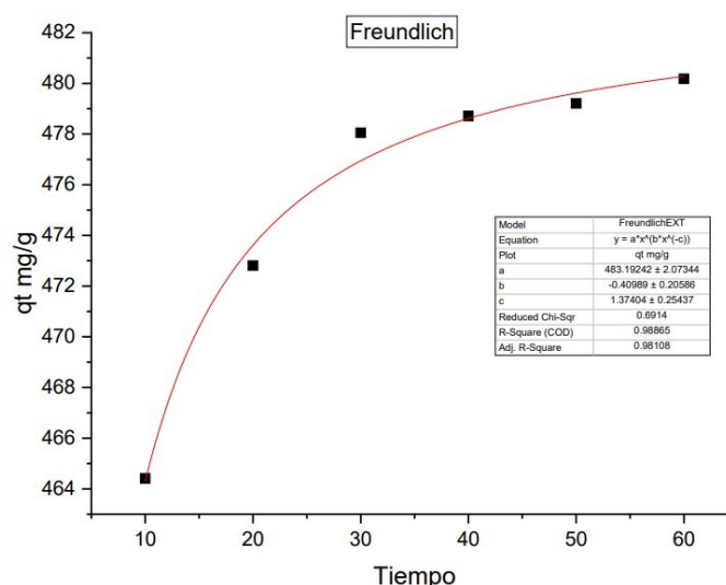
Gráfica 11. Modelo de Freundlich
