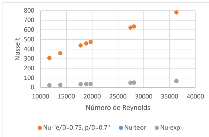
Figura 6. Numero de Nusselt ideal
