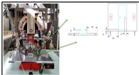
9. Propuesta de poka yoke , vista frontal y vista superior.
