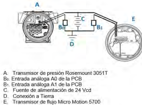
Figura 4. Diagrama de conexión de transmisores a PCB. Adaptado de [26].
